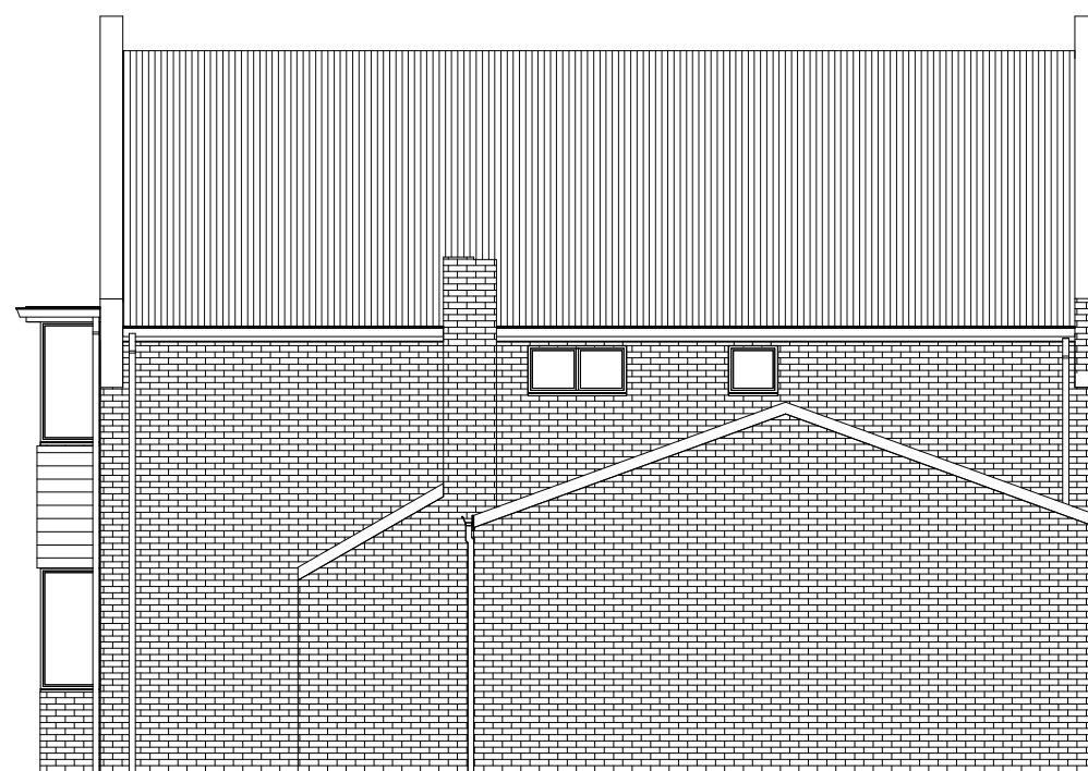
4 Side Elevation b-b 1 : 100
