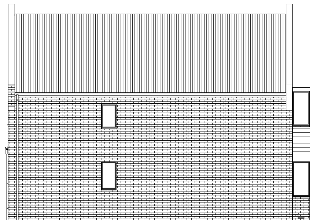
2 Side Elevation a-a 1 : 100
